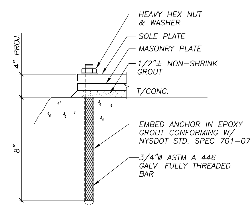
TYP. ANCHOR BOLT DETAIL N.T.S.
