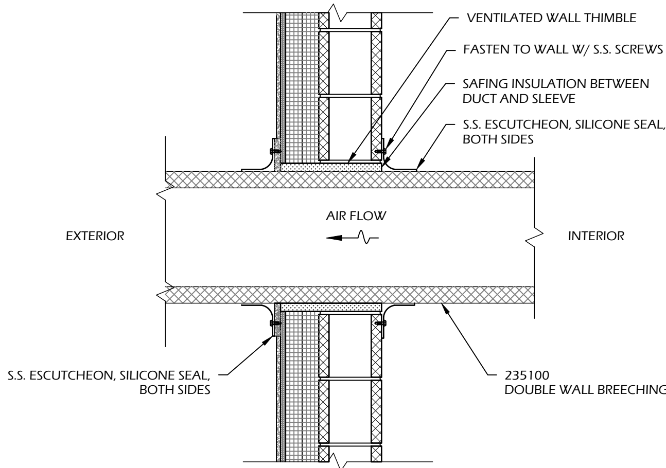
2 BREECHING/CHIMNEY PENETRATION THRU CMU WALL SCALE: N.T.S.
