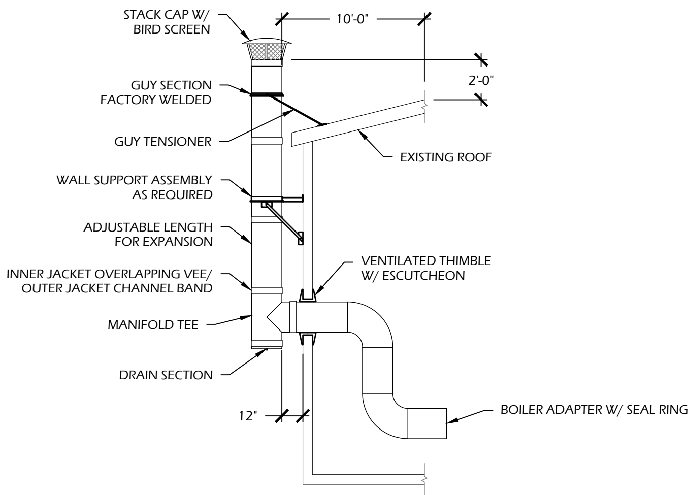
3 CHIMNEY STACK ELEVATION SCALE: N.T.S.
