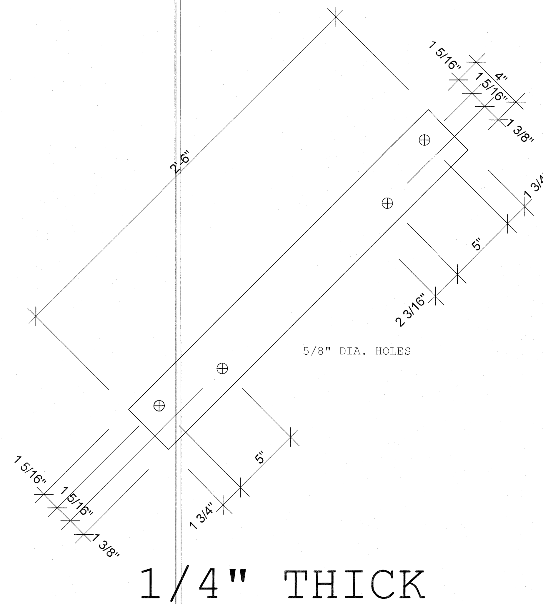
2 STEEL PLATE SCALE: 3" = 1'-0"
