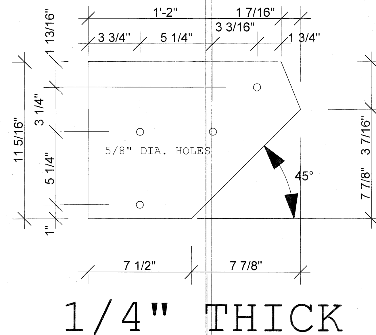
3 STEEL PLATE SCALE: 3" = 1'-0"
