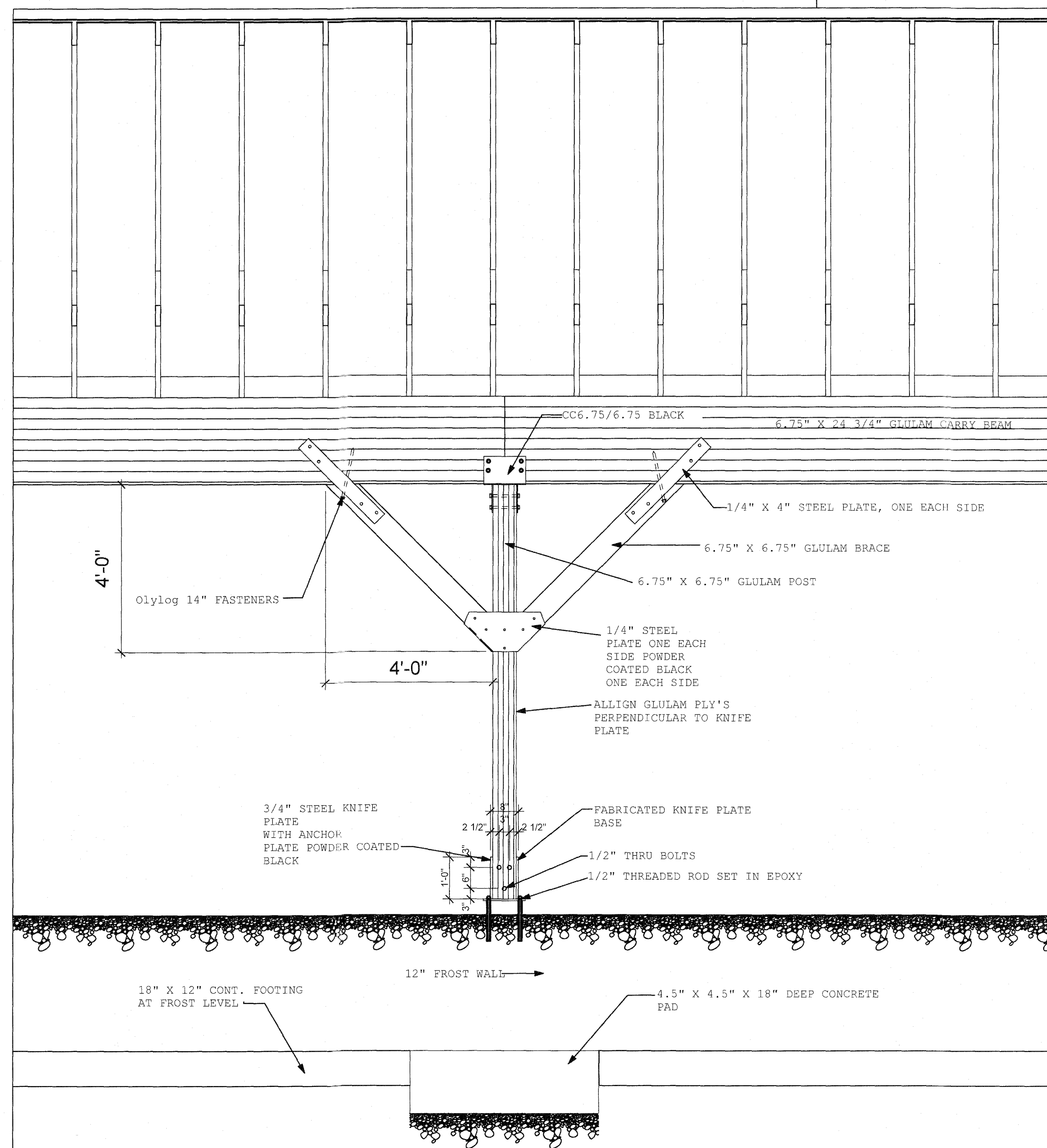
2 SECTION SCALE: 1/2" = 1'-0"
