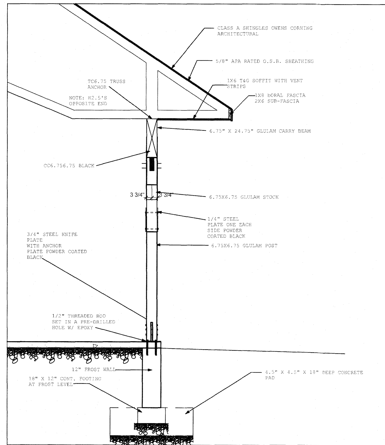
2 SECTION (1) SCALE: 3/8" = 1'-0"
