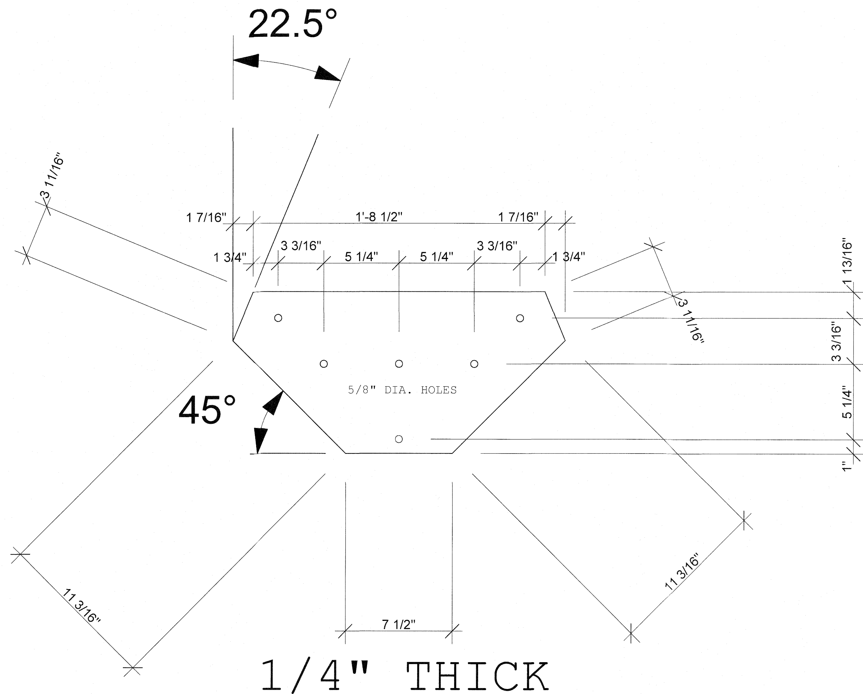
1 STEEL PLATE SCALE: 3" = 1'-0"
