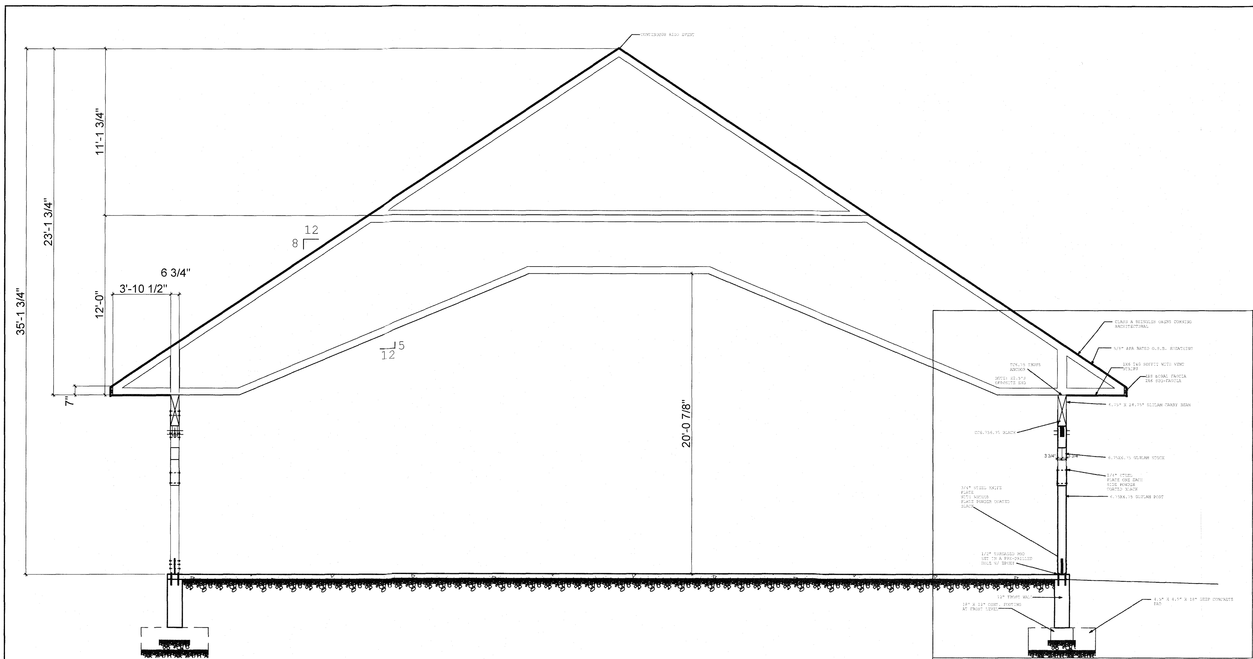
1 SECTION SCALE: 1/4" = 1'-0"
